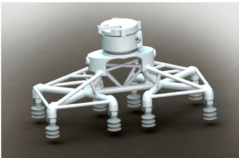
Leichtbau ermöglicht im Maschinenbau Einsparpotenziale, neue Gestaltungsmöglichkeiten und eine höhere Performance (Beispiel Greifer). (Quelle: Fraunhofer IPA/robomotion GmbH)
